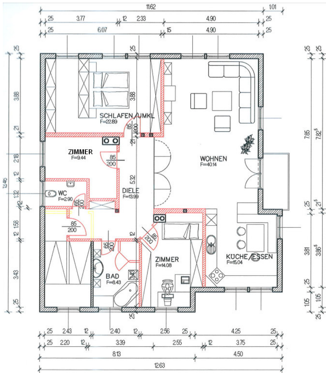
GRUNDRISS 1/100 DACHGESCHOSS
